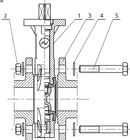
Схема монтажа
